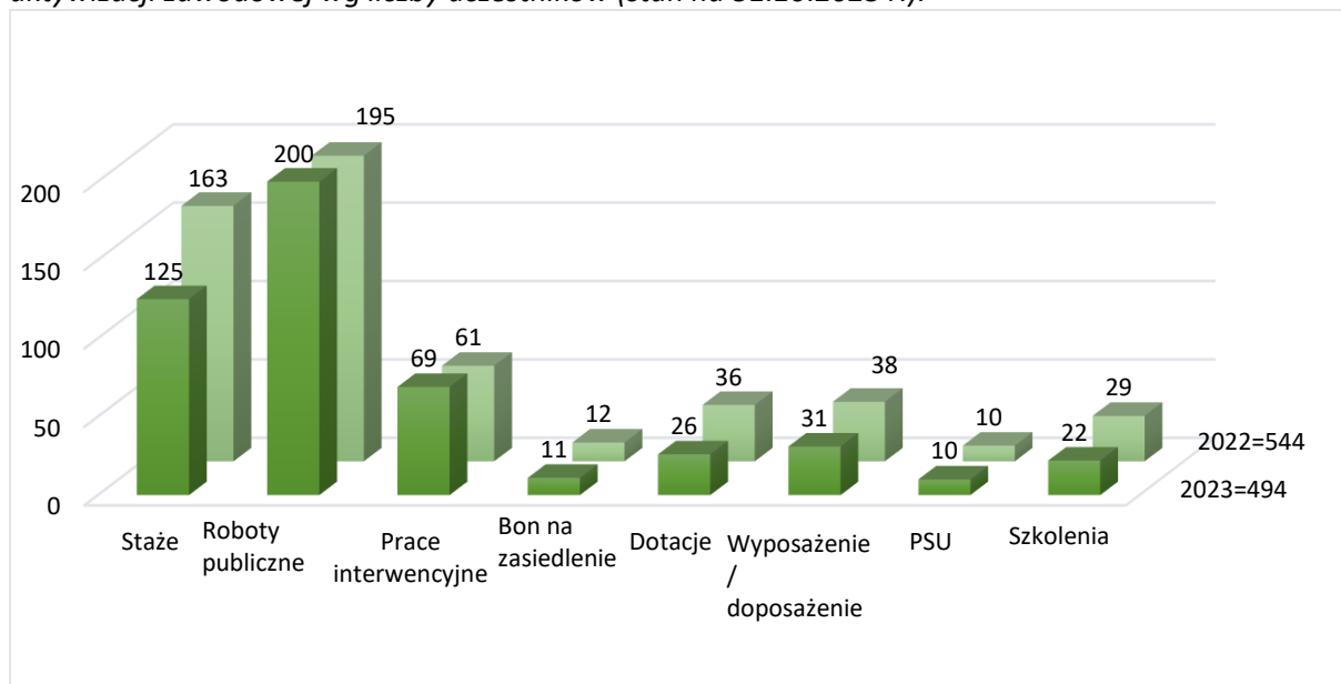
Wykres 4. Struktura zadań realizowanych w powiecie sokólskim w ramach podstawowych form aktywizacji zawodowej wg liczby uczestników (stan na 31.10.2023 r.).
